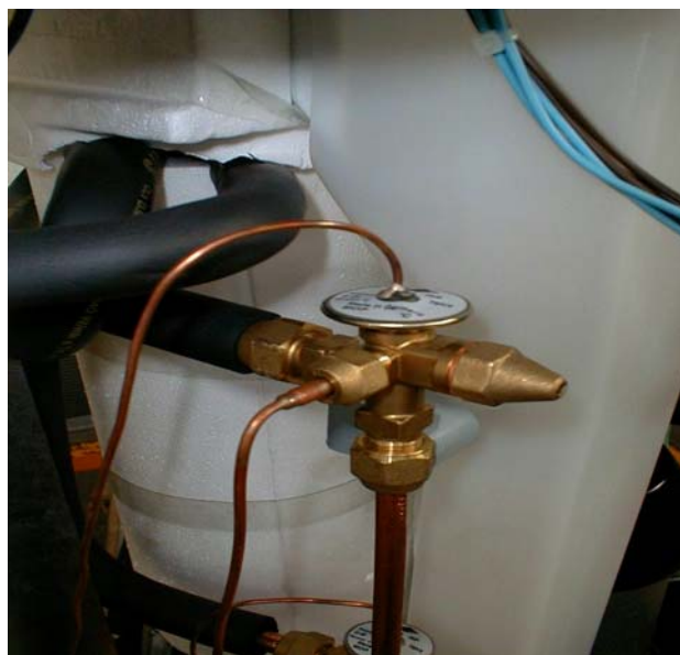
5 Valvola di regolazione della pressione di evaporazione costante (Danfoss KVP 12 nel MF 58 e Danfoss KVP 22 nel MF 68)
